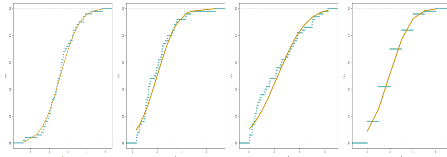
Şekil 2.1. ECDF plots
