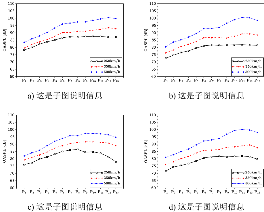
图 3-2 总声压级
